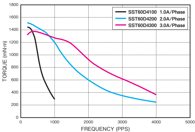
SST60D4XXX
