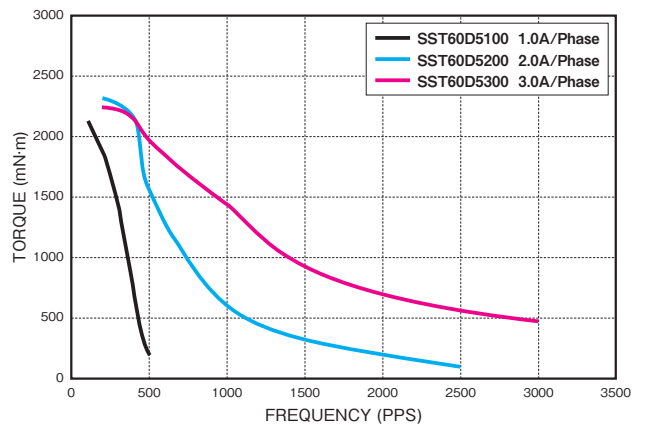
SST60D5XXX
