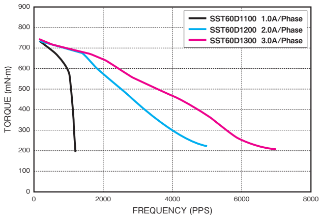
SST60D1XXX
