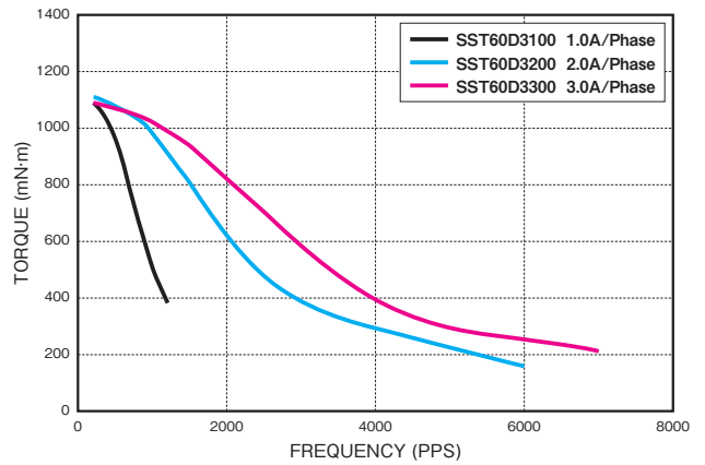
SST60D3XXX
